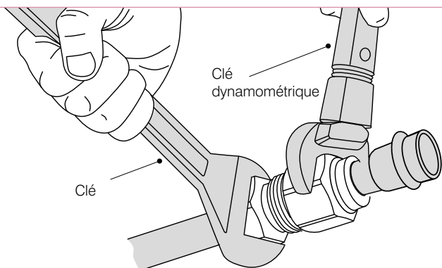
Serrer le raccord à l'aide d'une clé dynamométrique
